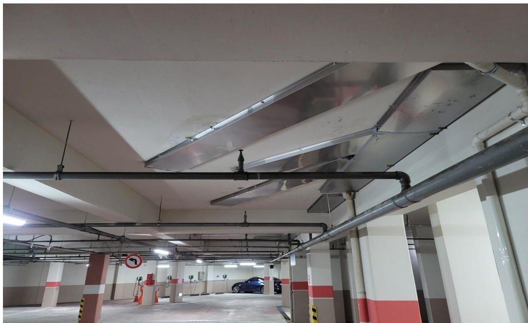
공사 후 : 유도배수 작업
