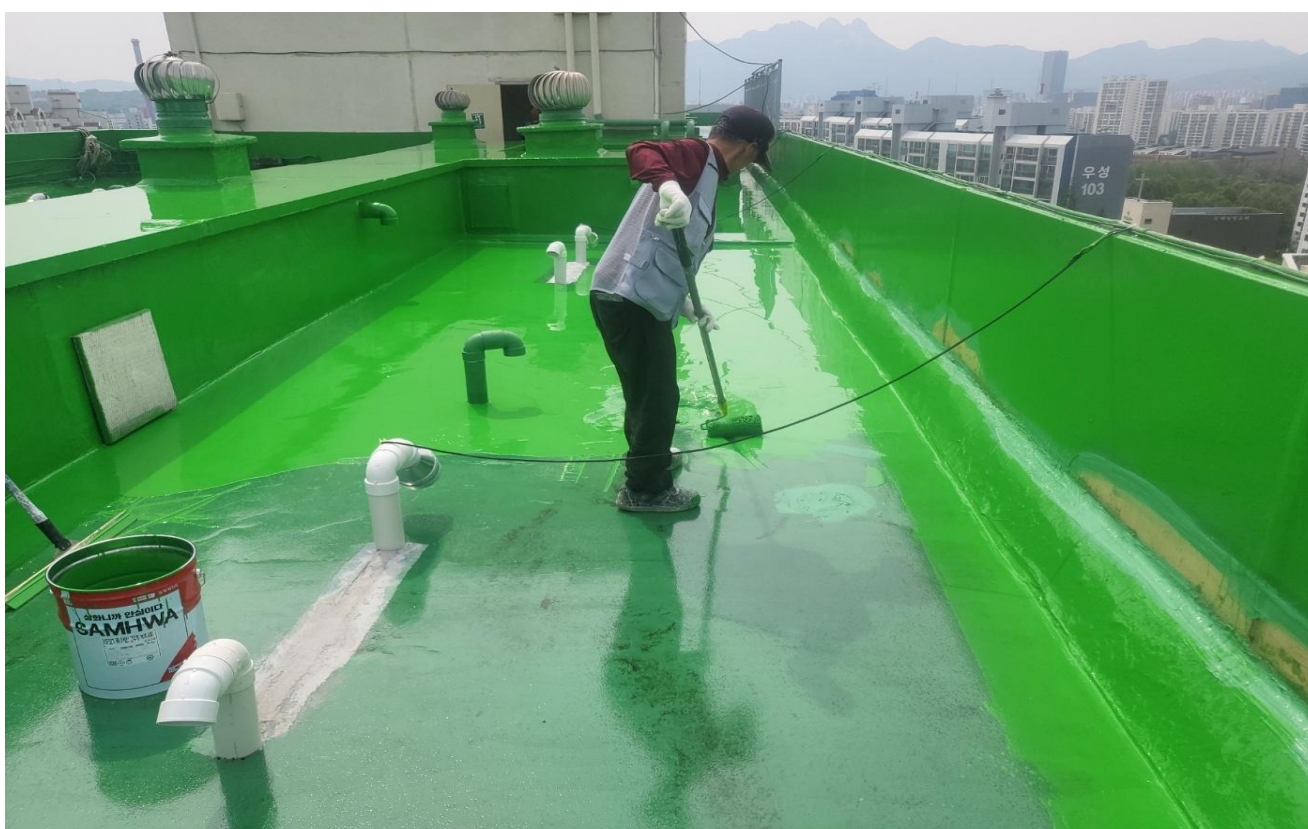
공사 중 (우레탄 중도 1차 도포)
