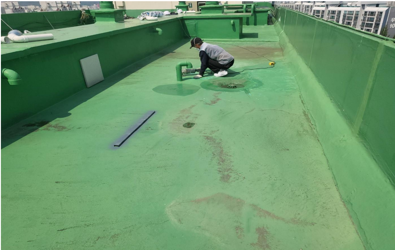
공사 중 (바탕면 정리)
