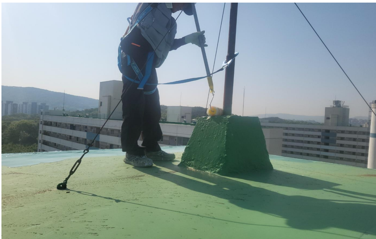
공사 중 (우레탄 하도 도포)
