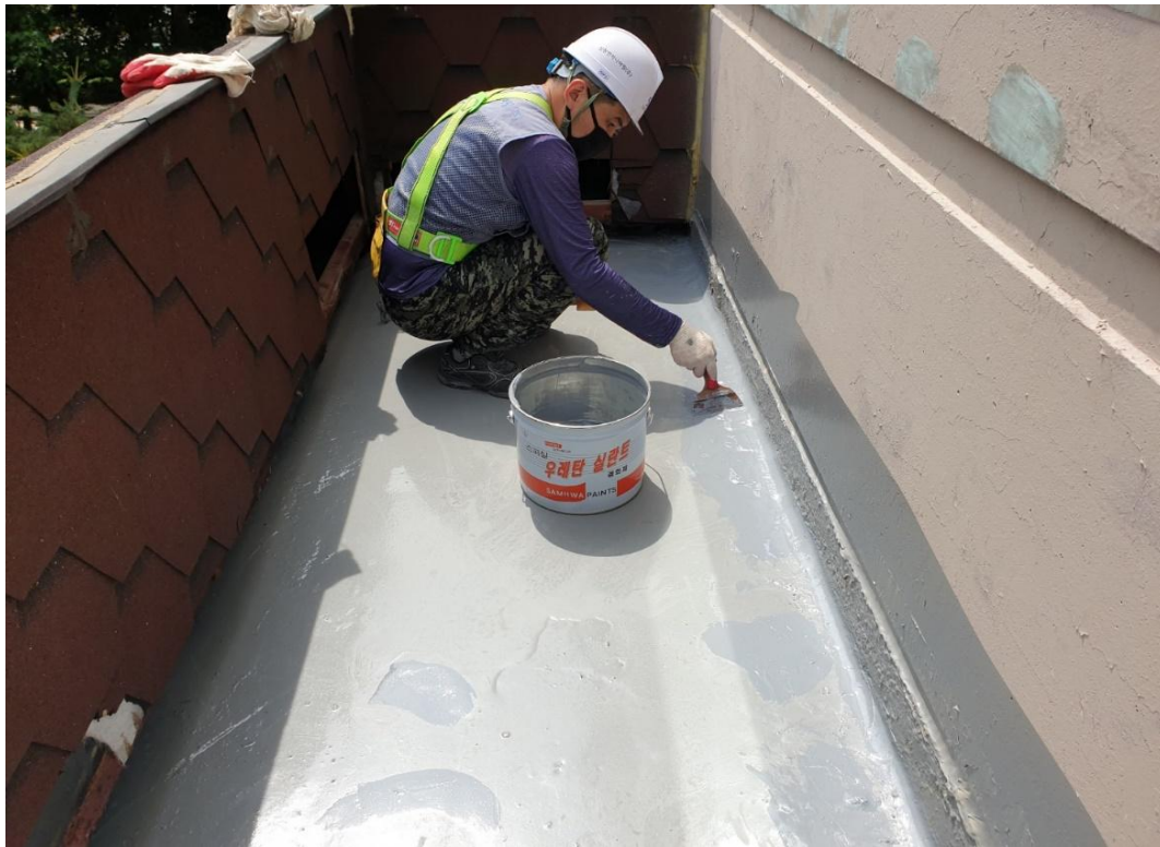
바닥보수작업 2차
