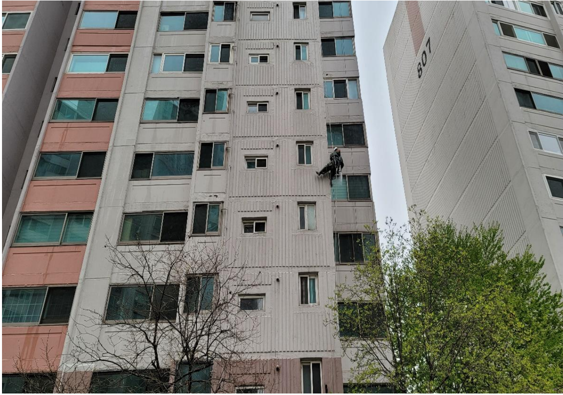
고압세척 공사중
