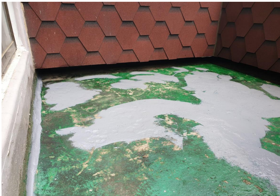
바닥 보수작업
