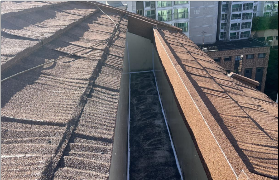
우레탄 실란트 시공
