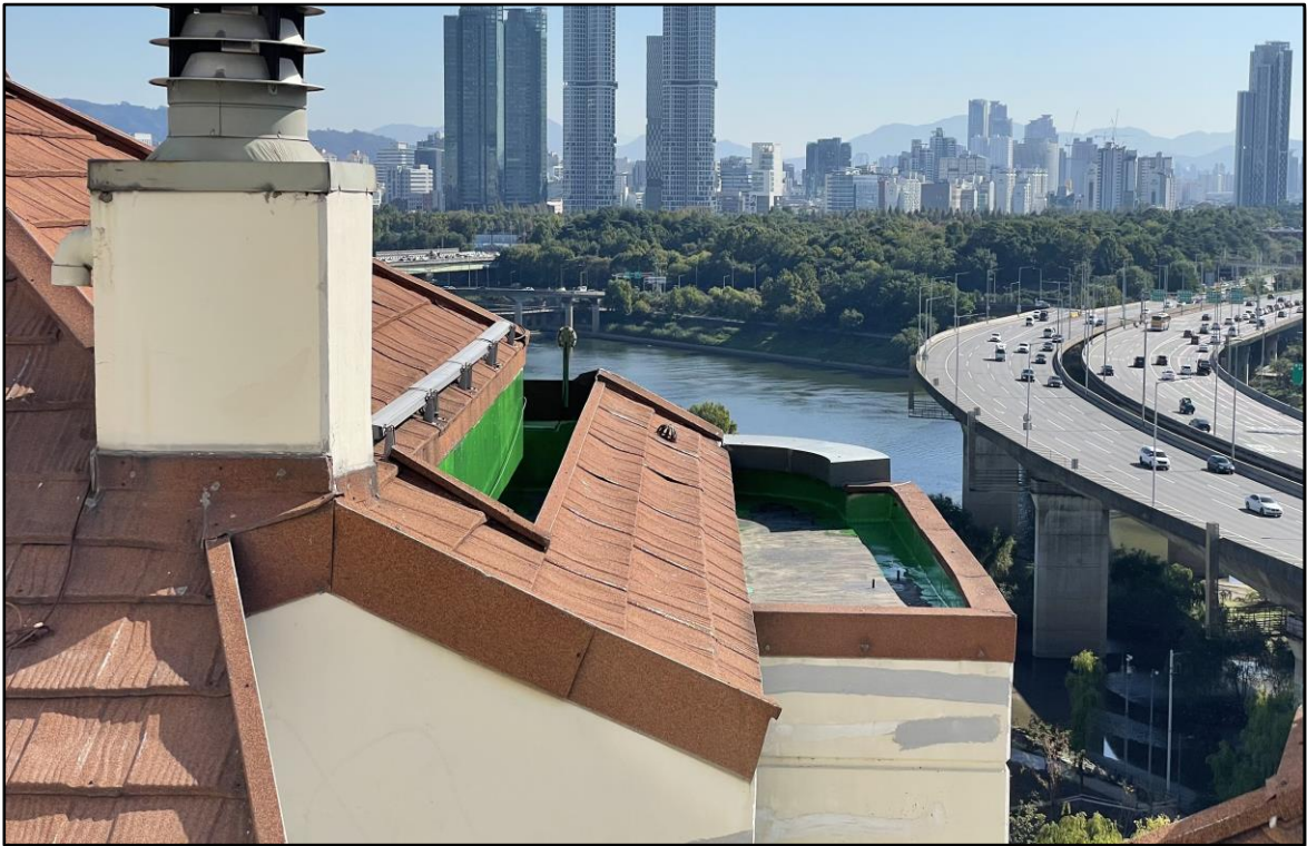
우레탄 중도 1차 시공
