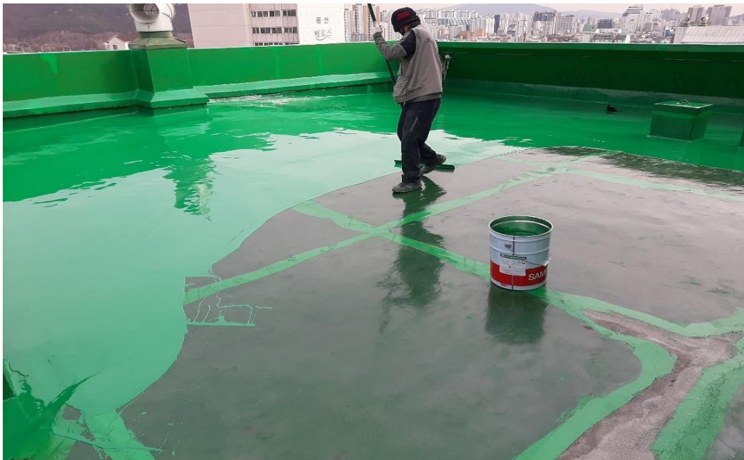
우레탄 중도 1차 도포
