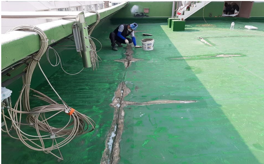
옥상 바닥 들뜸부위 콘크리트 몰탈보수
