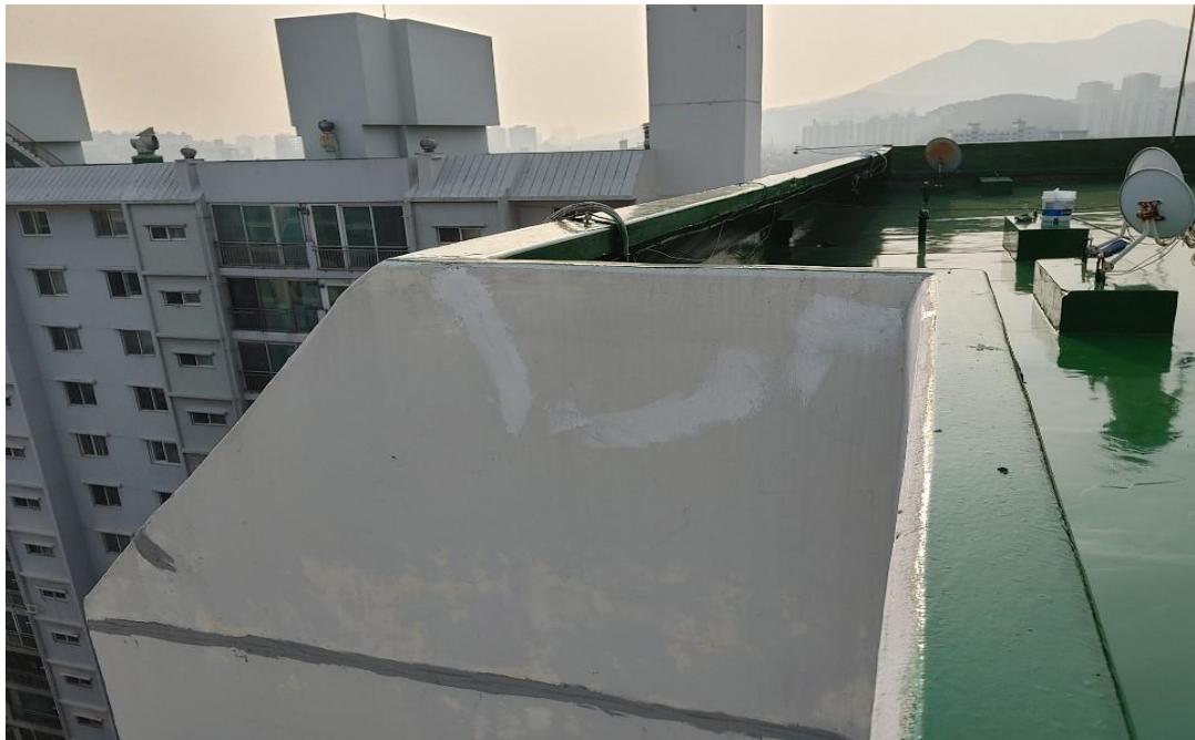
외벽 파라펫 균열보수
