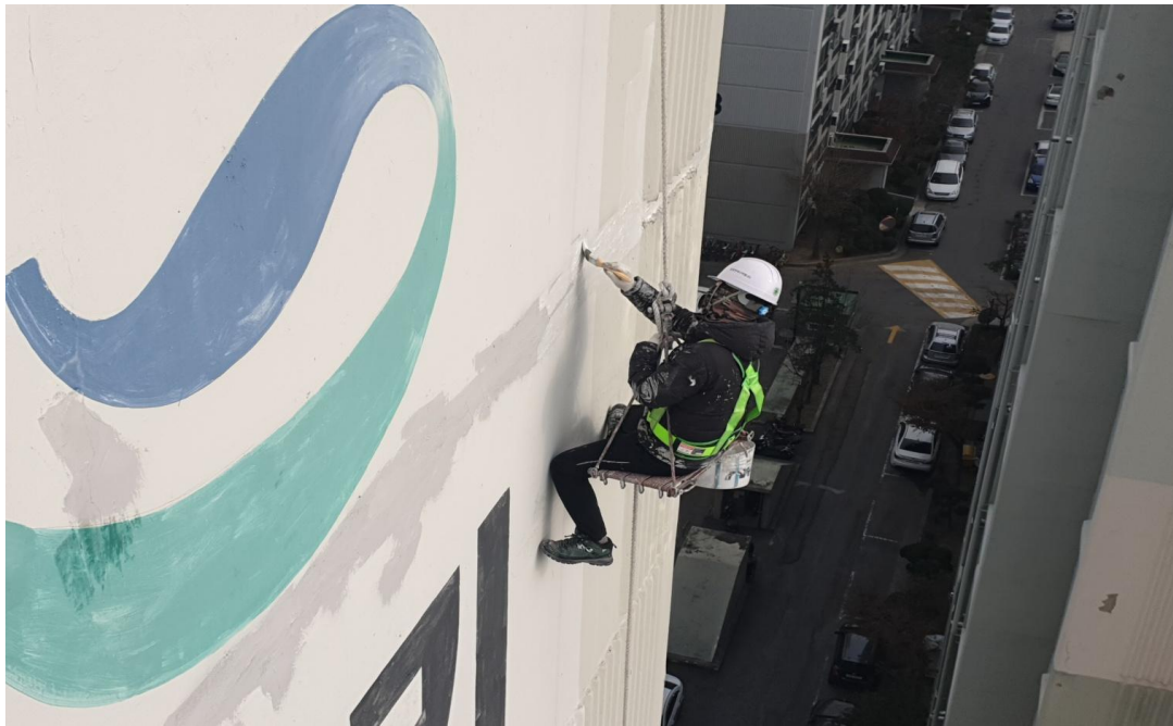
측벽 외벽 균열보수 후 도장마감(부분도장)
