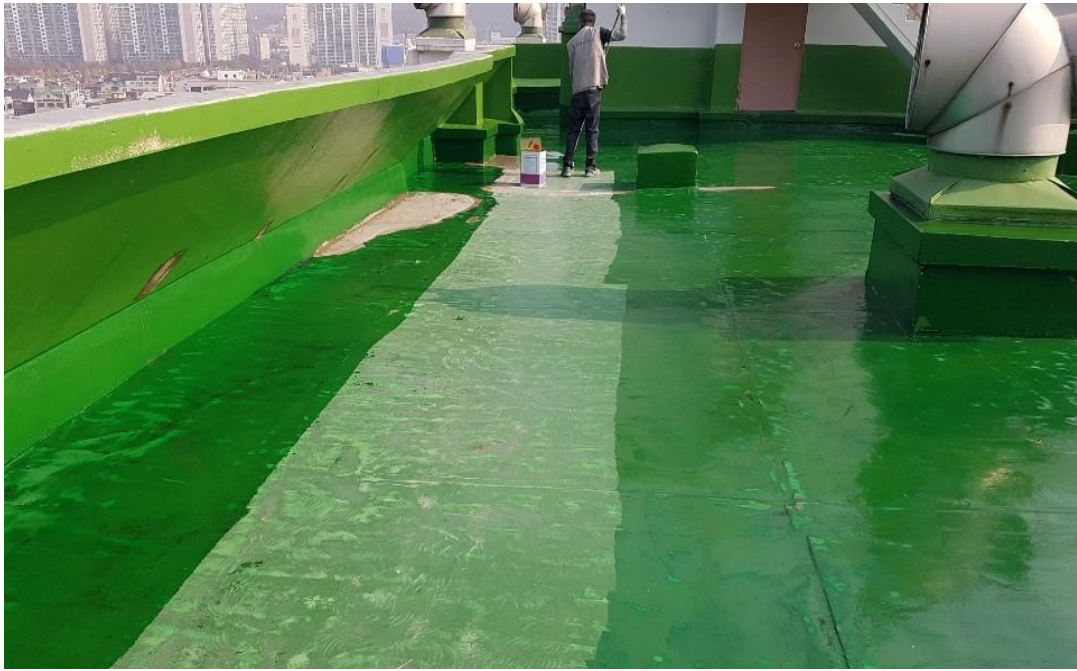
바닥 들뜸부위 보수 후 우레탄 프라이마 도포
