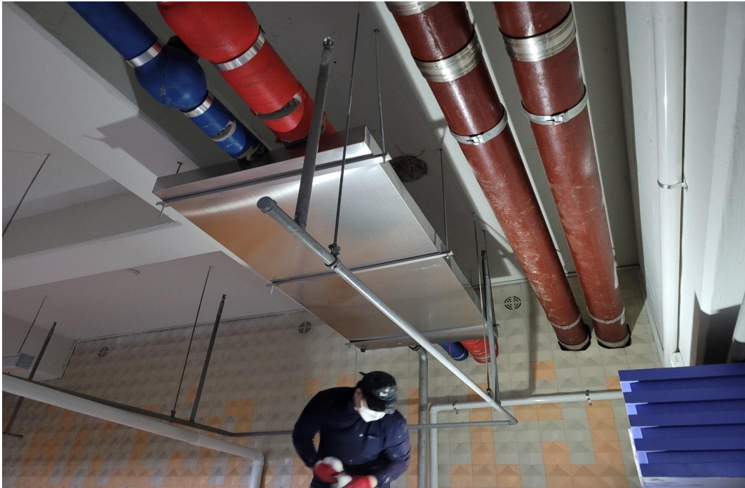
지하주차장 천장 누수부위 유도보수 공사 중
