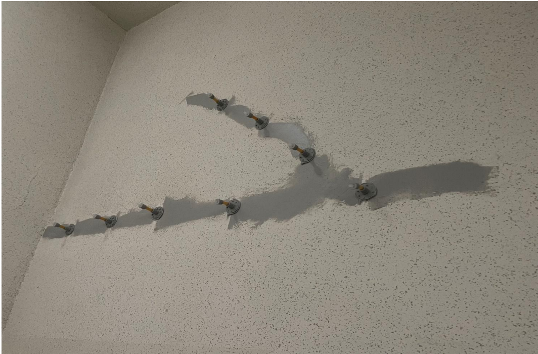
공용계단실 대균열 T-PORT 주사기 주입 시공 중
