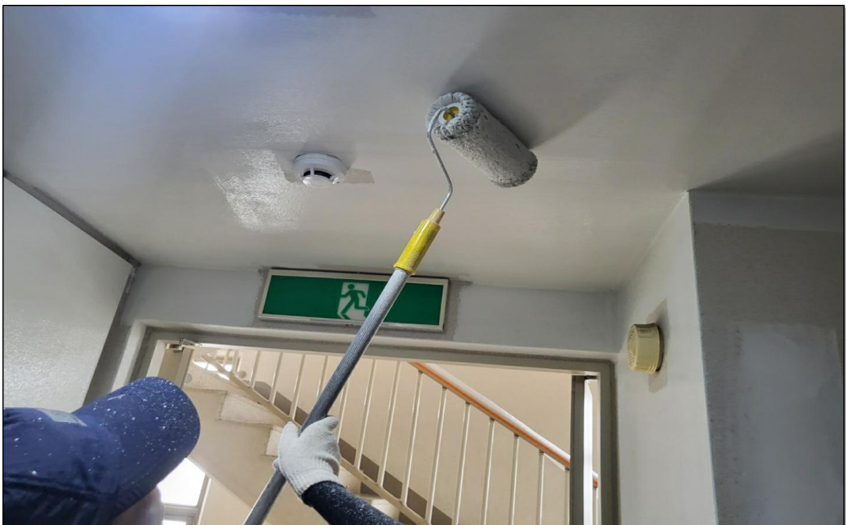
공용계단실 내부 수성페인트 도장
