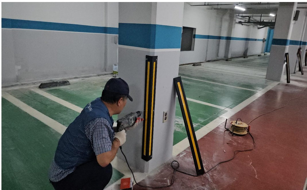
공사 중 (코너 비트 설치)
