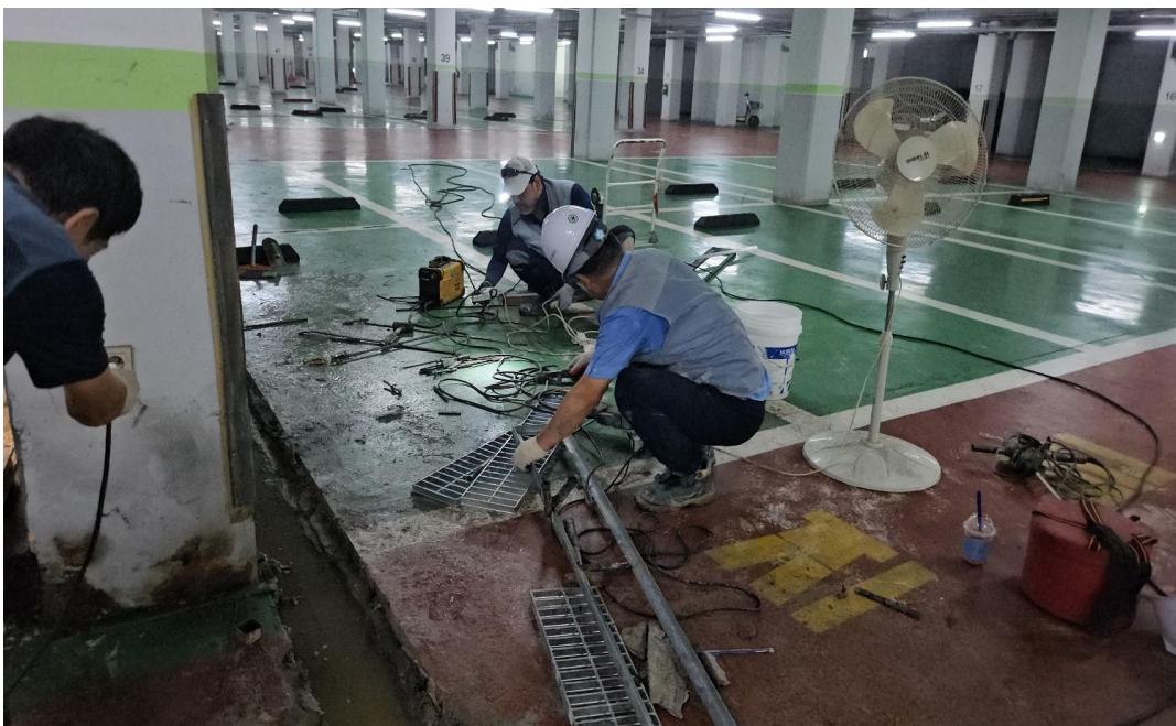
공사 중 (코너 비트)
