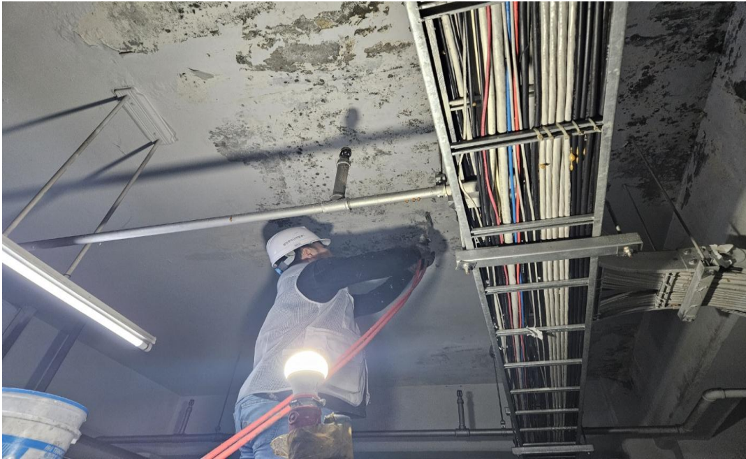
공사 중 (인젝션 주입)
