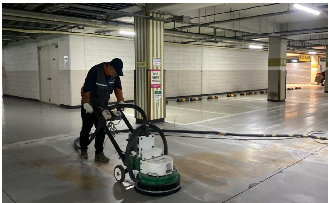
공사 중 (바탕면 정리)
