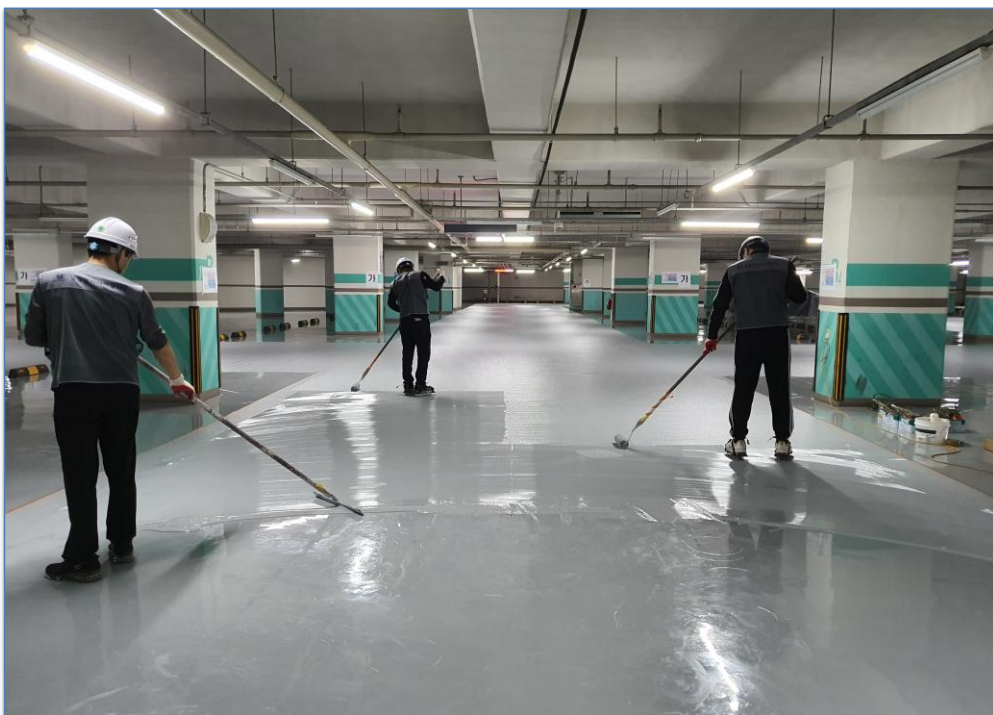
에폭시 엠보 도포 작업
