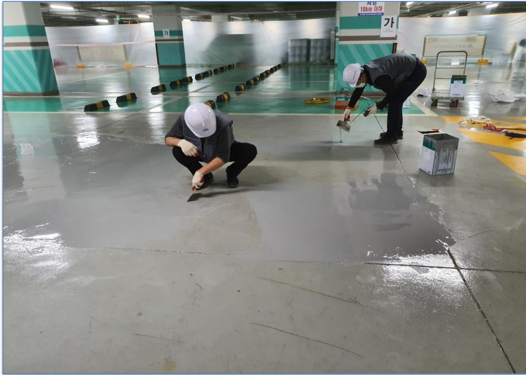
바닥 단면복구 작업
