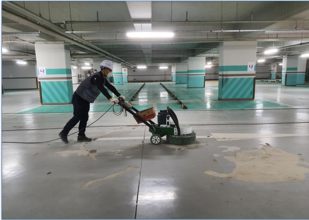
바닥 바탕면 정리 및 스크래치 작업
