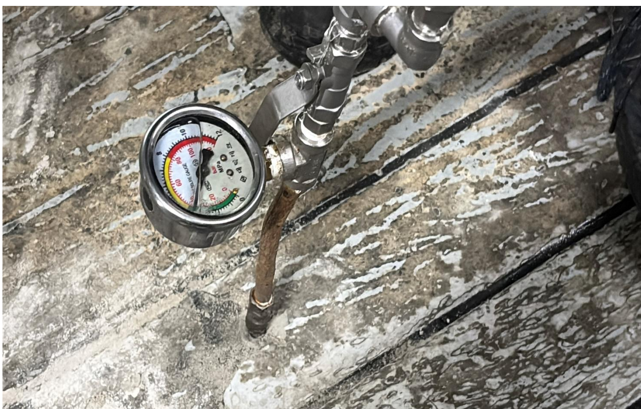
공사 중 (배면 그라우팅)
