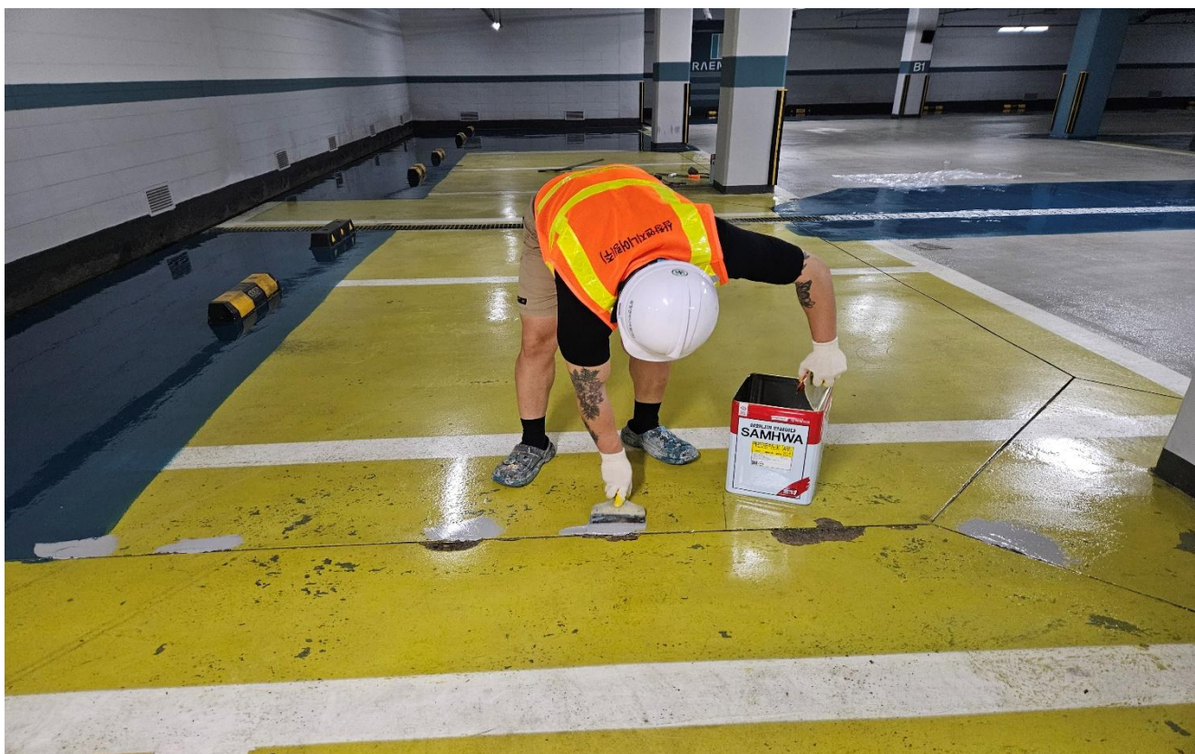
공사 중 (바닥 균열보수)
