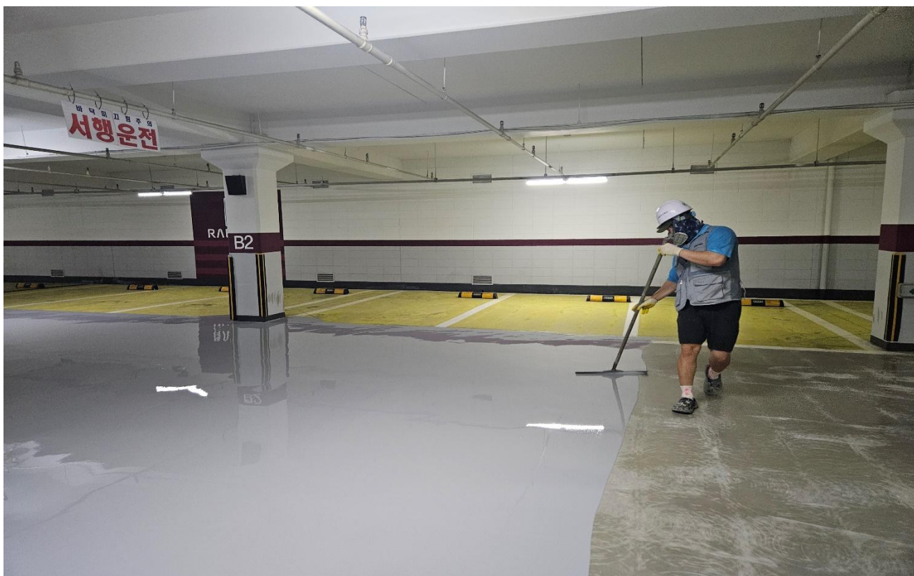
공사 중 (에폭시 중도 도포)
