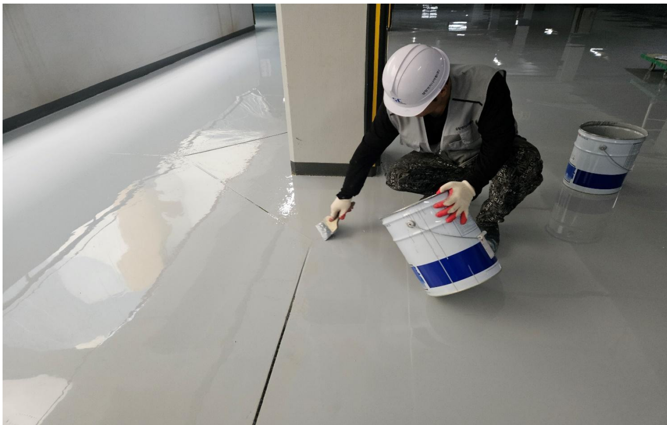
공사 중 (바닥 균열보수)
