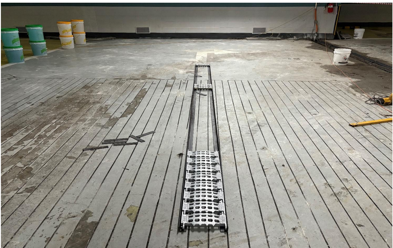
공사 중 (무소음 트렌치)
