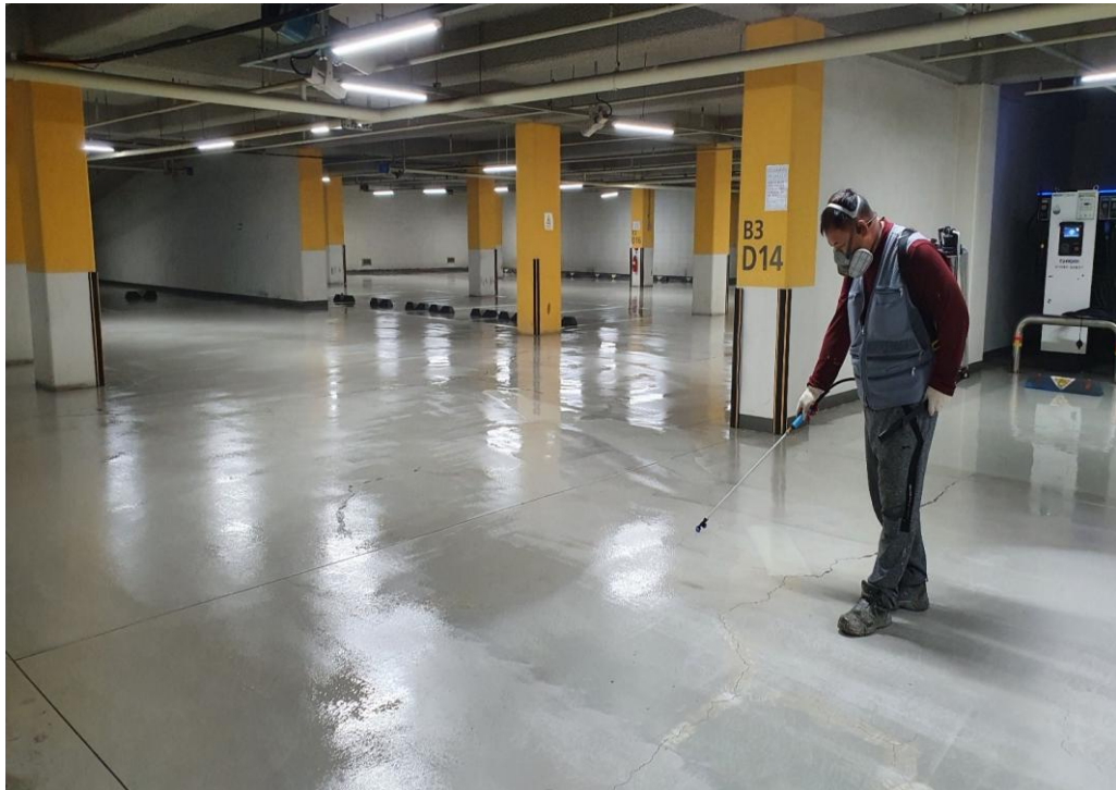
에폭시 프라이머 도포
