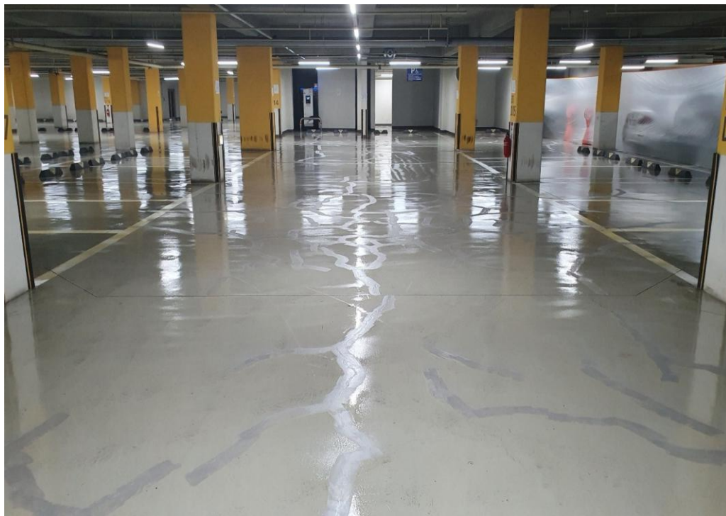
에폭시 퍼티 시공-균열보수
