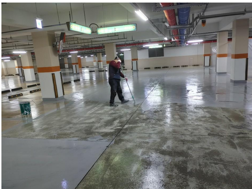
지하주차장 바닥 에폭시 도장-주행로 에폭시 라이닝 1차 도포
