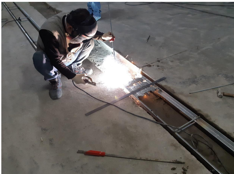
무소음트랜치 설치-앵글 용접
