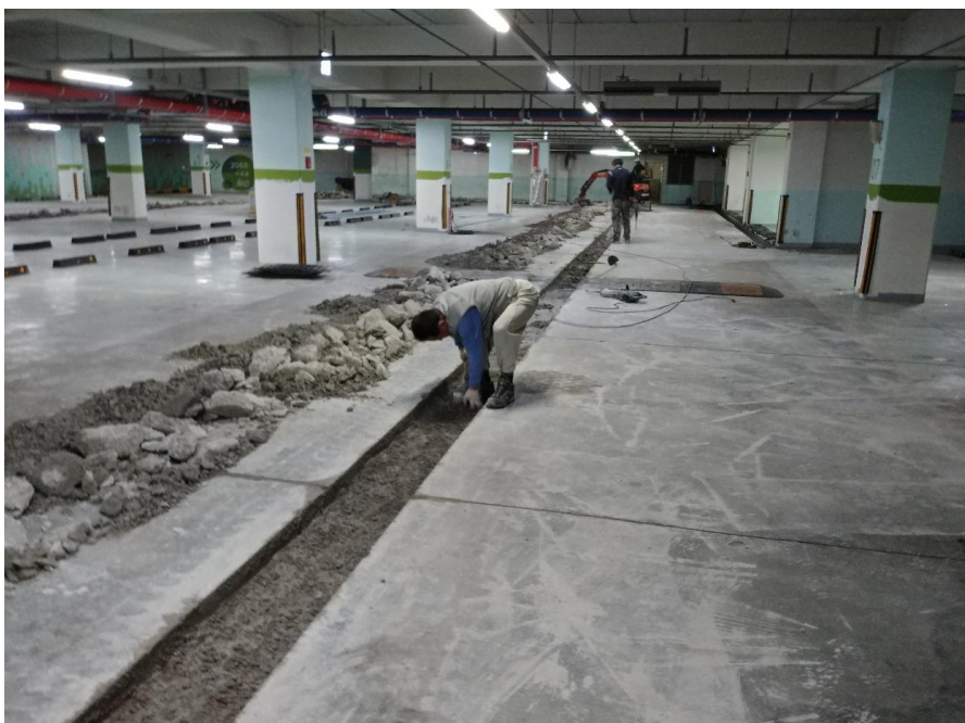
무소음트랜치 설치-바닥 파쇄
