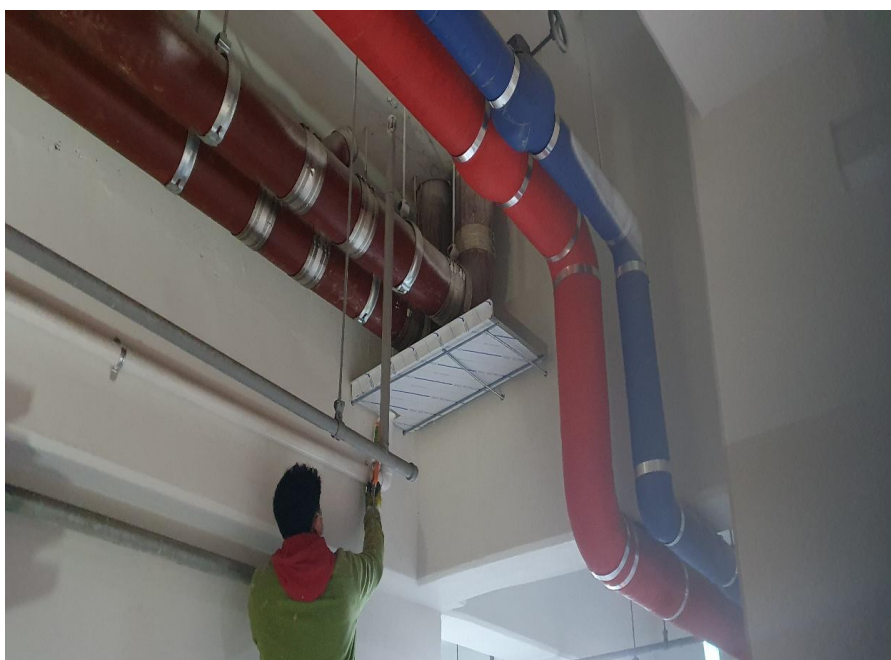
지하주차장 천장 누수보수-유도판 부착
