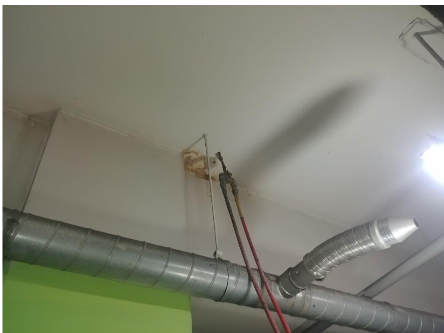
지하주차장 천장 누수보수-아크릴 주입
