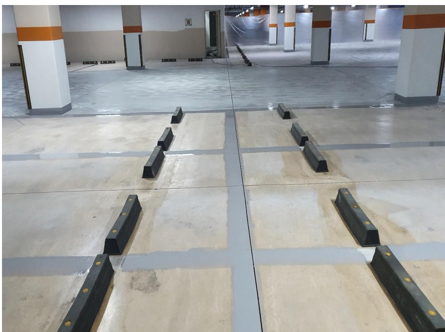
지하주차장 바닥 에폭시 도장-주차선 에폭시 라이닝 도포
