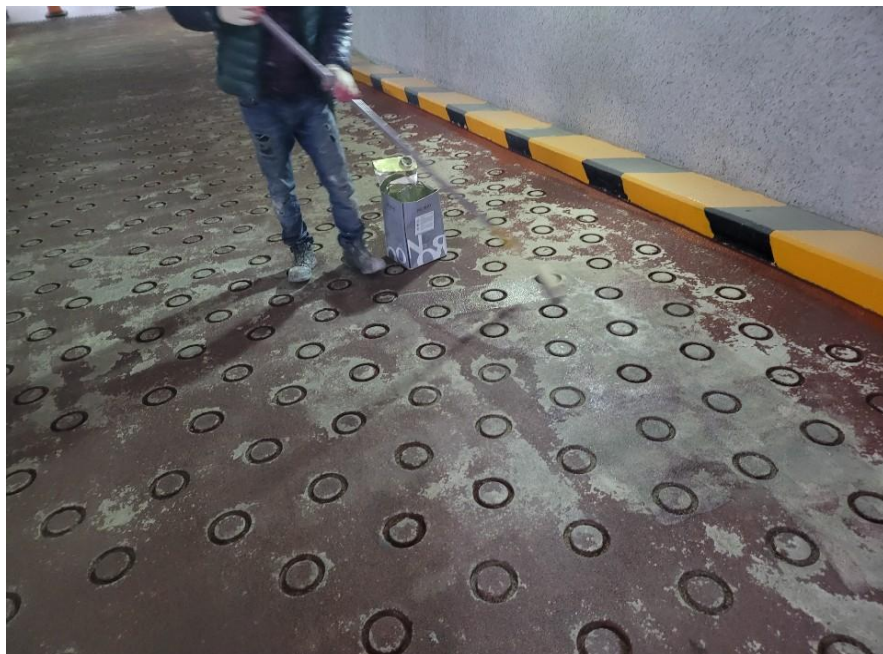
지하주차장 바닥 에폭시 도장-램프 바닥 에폭시 상도도장
