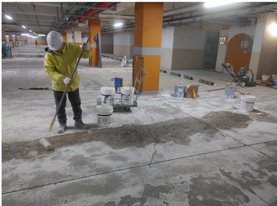
지하주차장 바닥 에폭시 도장-부실부위 표면강화제 도포
