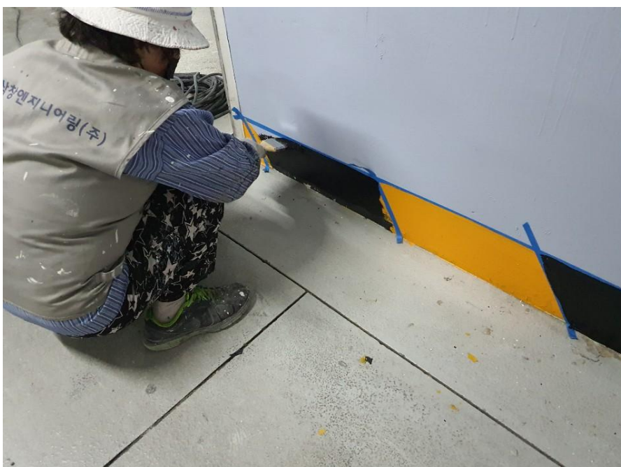
지하주차장 내부 도장-연석 안전페인트 도장
