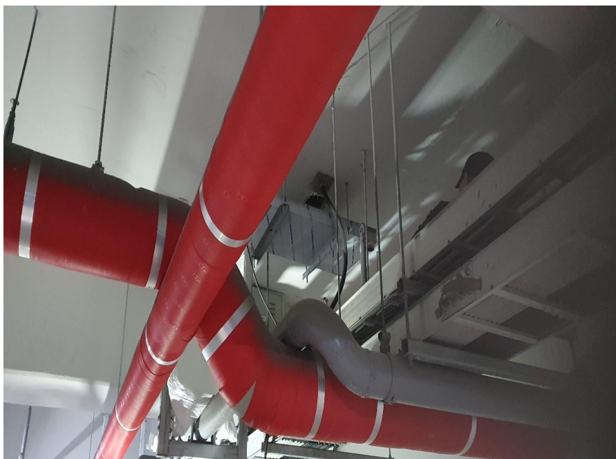
지하주차장 천장 누수보수-유도판 부착
