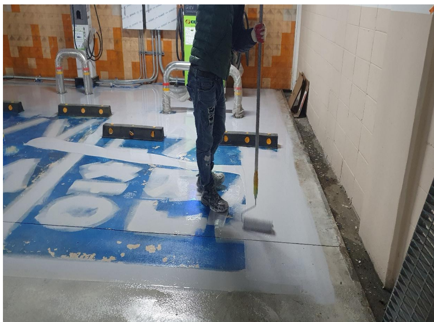
지하주차장 바닥 에폭시 도장-주차면 에폭시 상도 1차코팅
