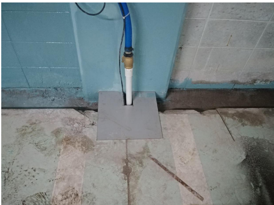
집수정 설치-배수펌프 설치
