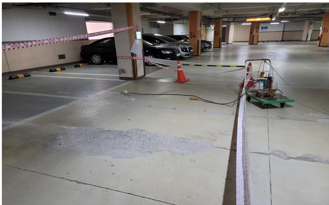
대균열 고점도 주입제 주입중(T-port 공법)
