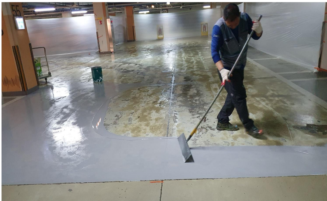
에폭시 라이닝 1차 도포 중
