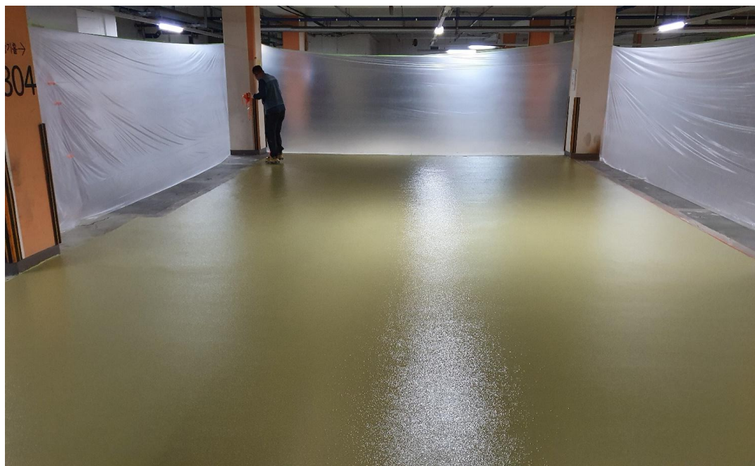
에폭시 엠보 도포 중
